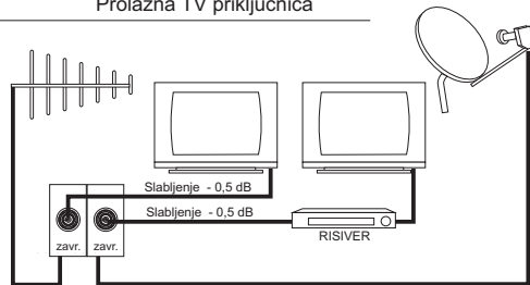
Primer povezivanja dve završne priključnice
