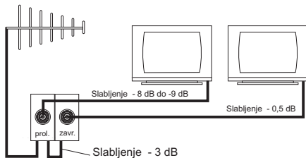
Primer povezivanja prolazne i završne priključnice
