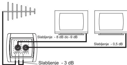
TV priključnica sa dva modula (prolazno/završna)
