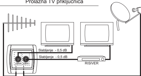
TV priključnica sa dva modula (završno/završna)
