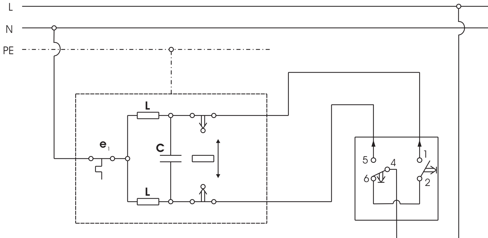
Motor sa bimetalnom zaštitom i krajnjim mikro-sklopkama
